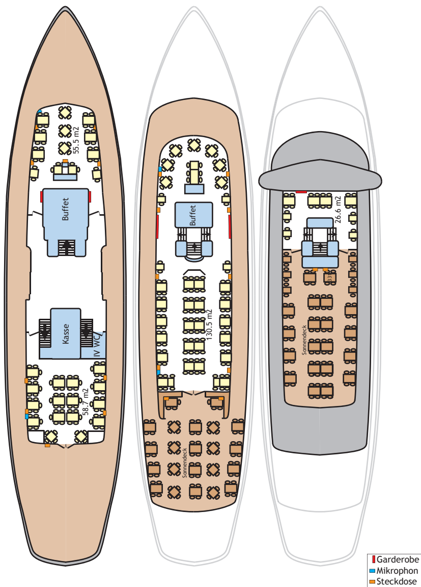
Hauptdeck
