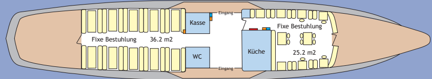
Hauptdeck
